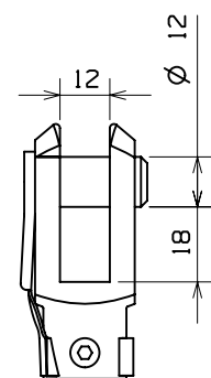
DETAIL BELIERE Echelle 1:2
