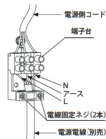
図 1 【端子台への接続】
