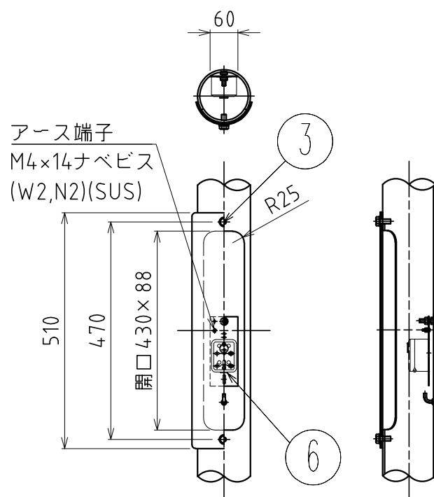
開口部詳細
