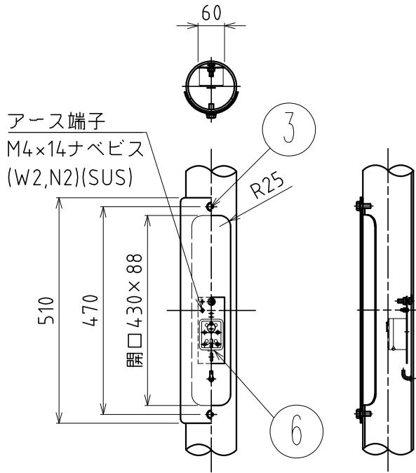
開口部詳細
