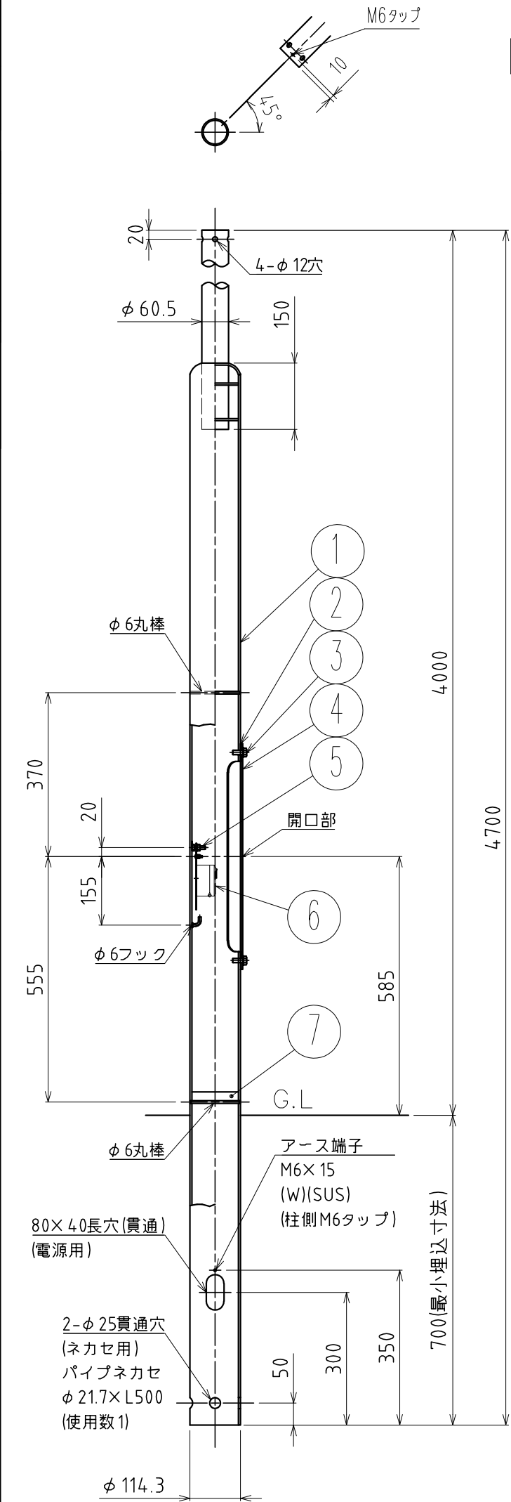
ポール全体図
