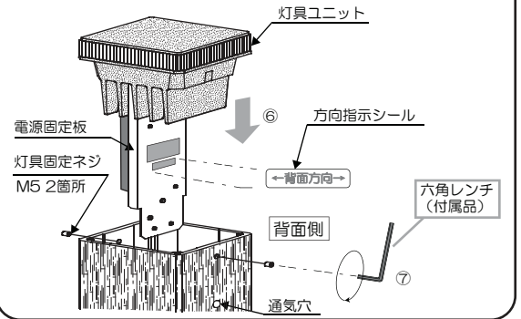
(図3) 器具内配線の接続と取付 <図はH-304G・H>
