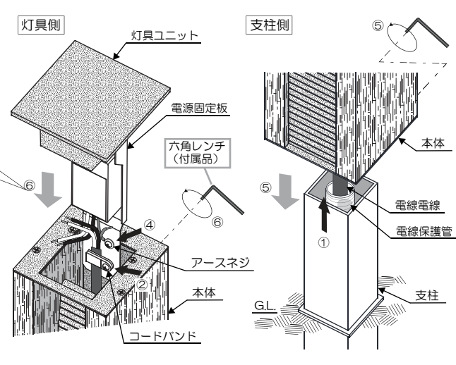
(図2) 器具内配線の接続と取付 <図はH-302G・H>
