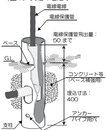
(図1) 支柱の埋込み
