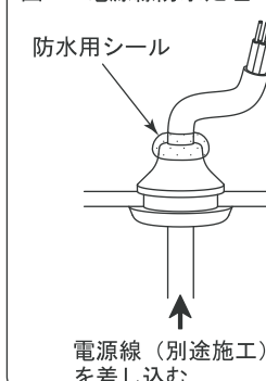
図 7 電源線防水処理
