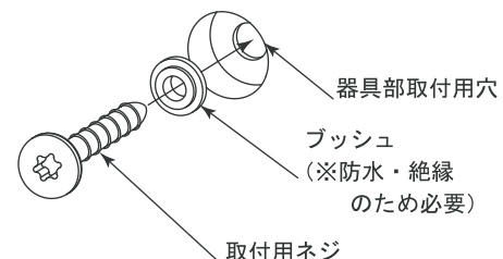
図 3 取付ネジの注意
