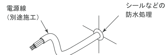
図 4 電源線入り口の処理
