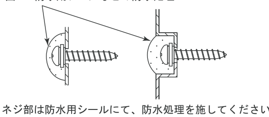
図 5 防水用シールなどの防水処理
