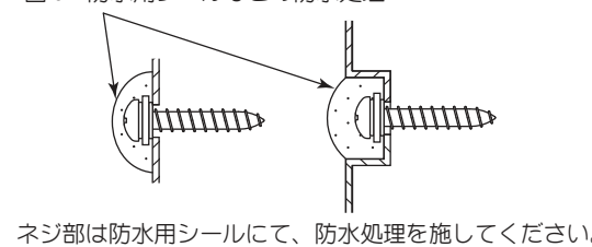
図6 防水用シールなどの防水処理
