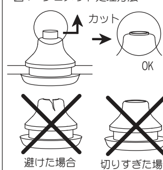
図7 グロメット処理方法
