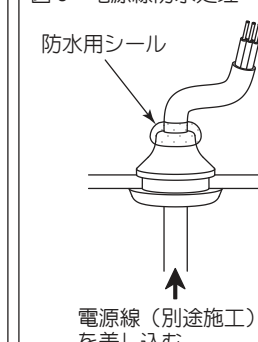
図8 電源線防水処理
