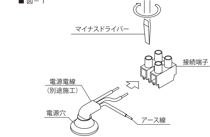
■ 取付方向(器具正面から見た図)
