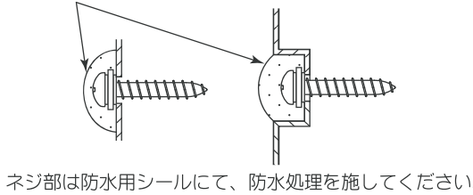
図2 防水用シールなどの防水処理
