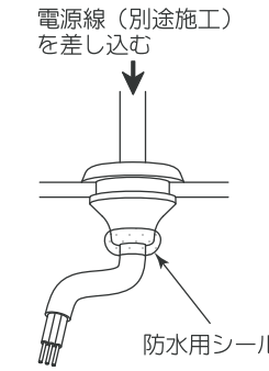
図4 電源線防水処理
