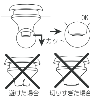
図3 グロメット処理方法
