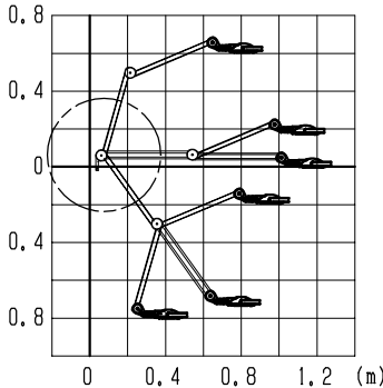
(m) アームの可動範囲図
