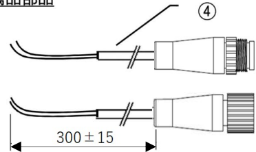
付属品部品
