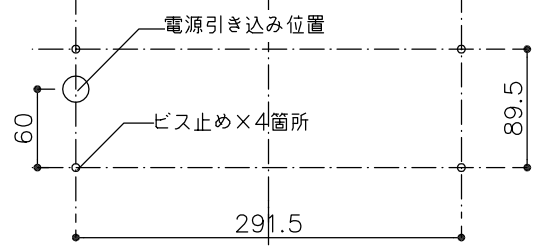
電源BOX直付け時
