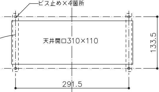
電源BOX埋込み時
