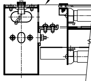
連結部詳細図
