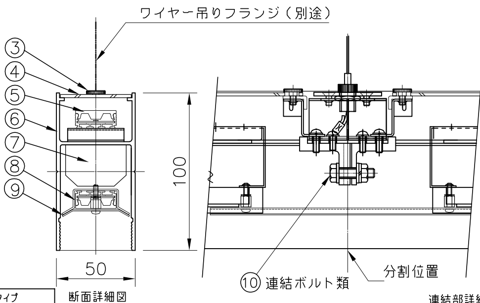
連結部詳細図
