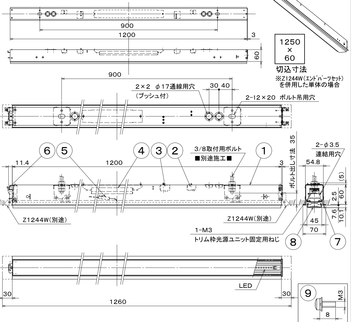
全体図
