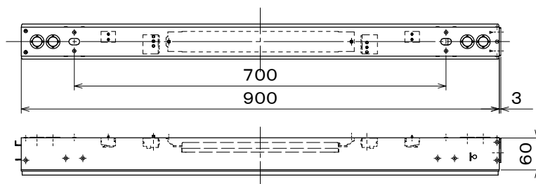
全体図
