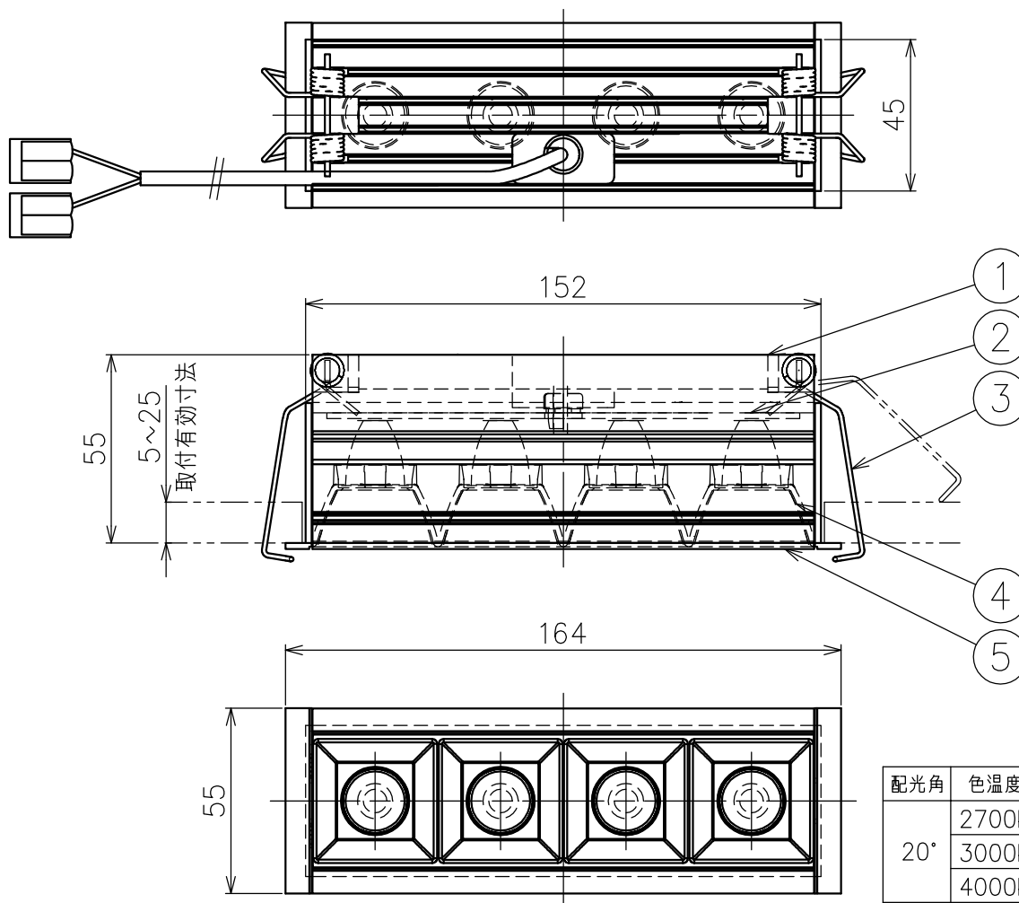
切込寸法
