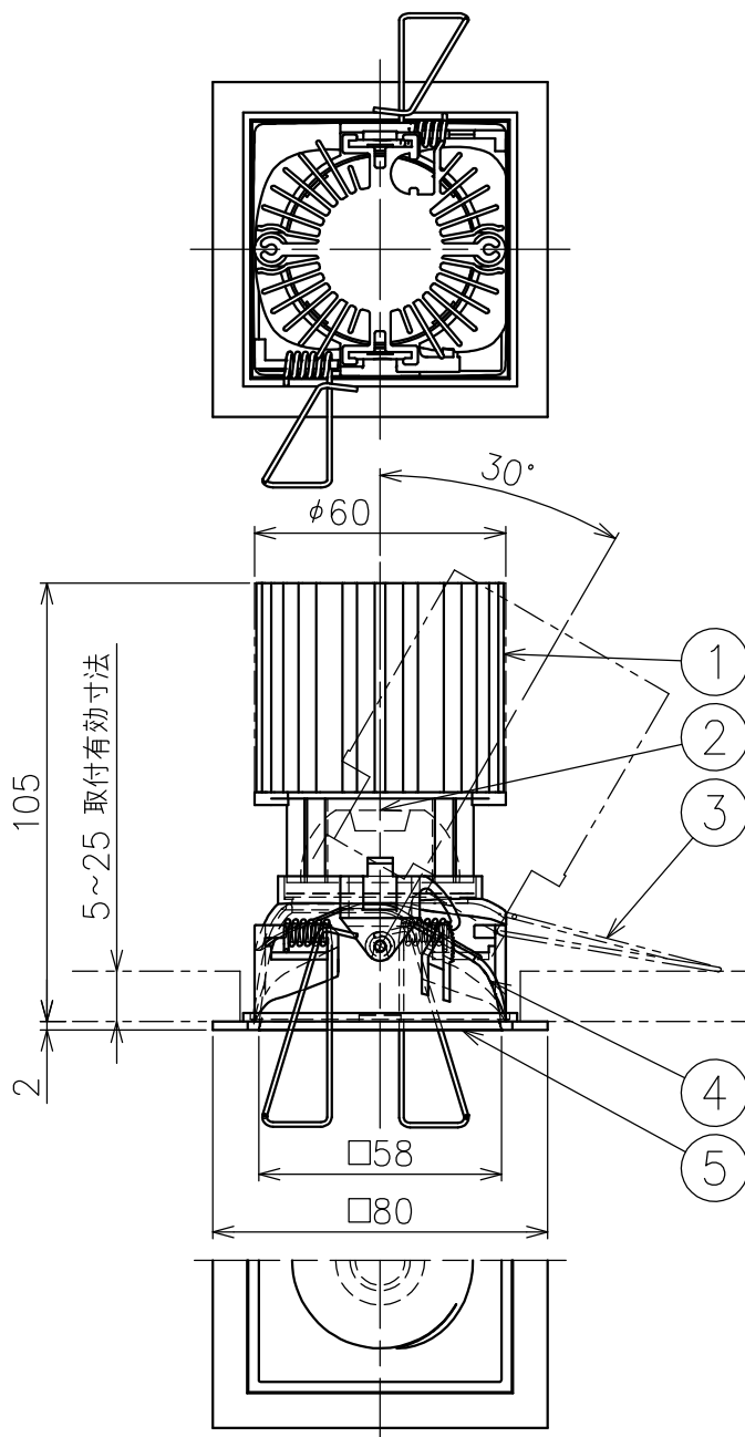
切込寸法
