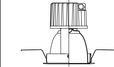
断面
