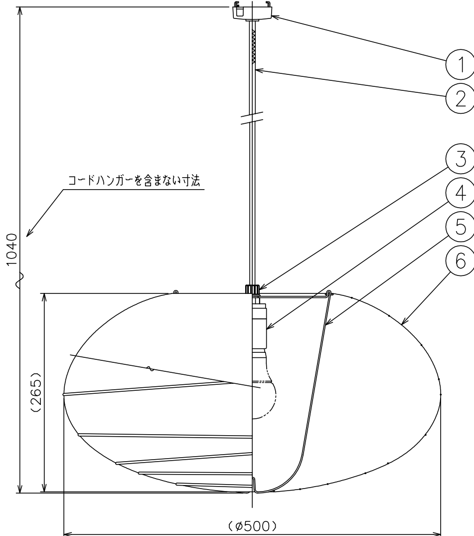
角型引掛シーリング
