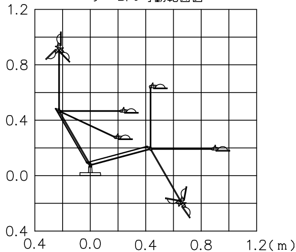
アームの可動範囲図
