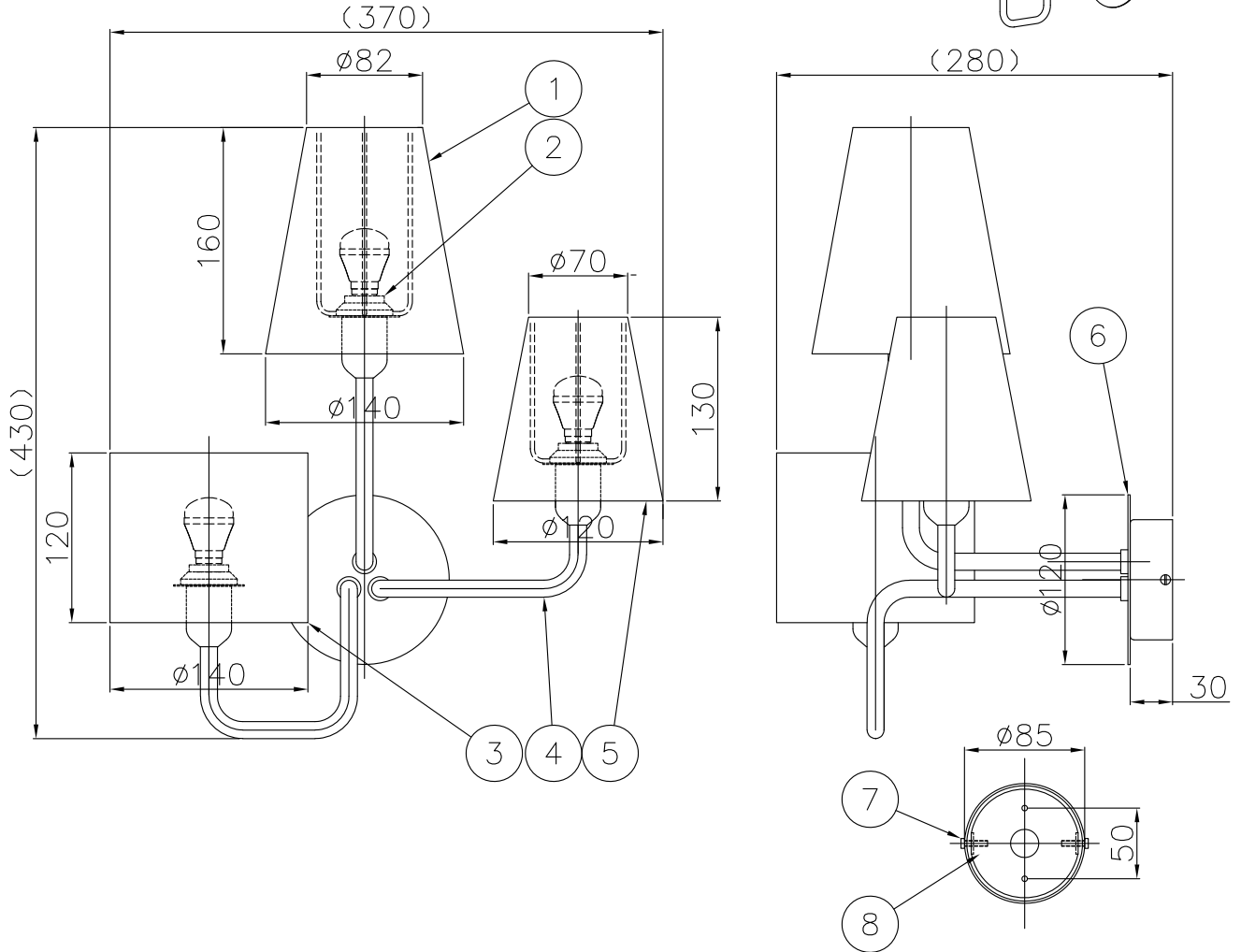
取付部詳細
