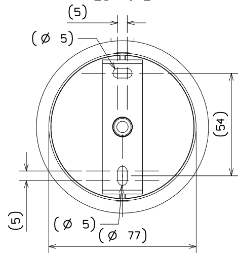
Detail systeme de fixation Ech 1:2
