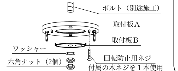
角型引掛シーリング
