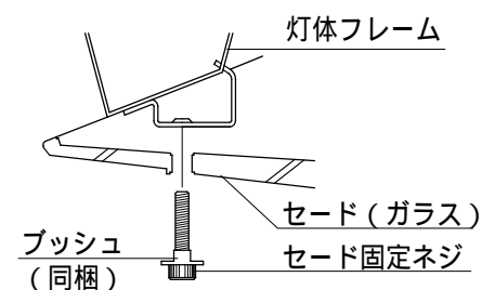
図1) セード (ガラス) 固定方法 断面図
