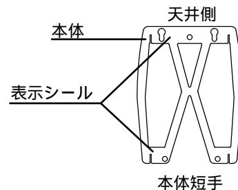
本体短手
