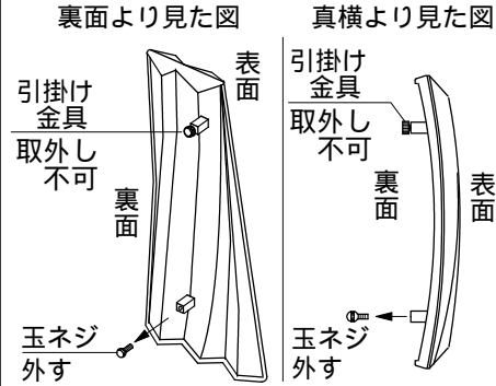
真横より見た図
