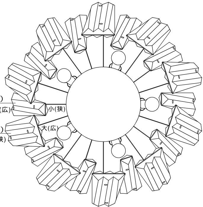
器具を下より見た図
