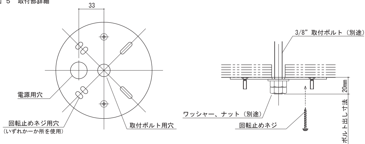
図 5 取付部詳細
