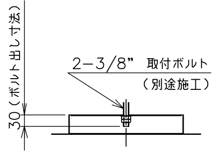
取付部詳細
