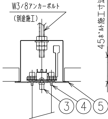
吊元詳細図S1/5
