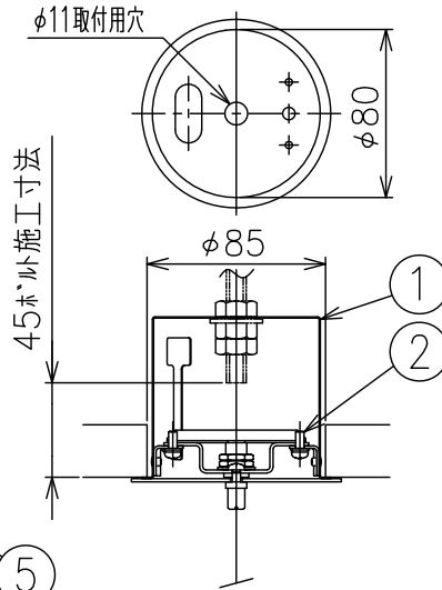
吊元詳細図S1/5
